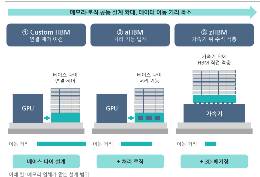
그림 38. 베이스 다이 기능 확장의 3단계
