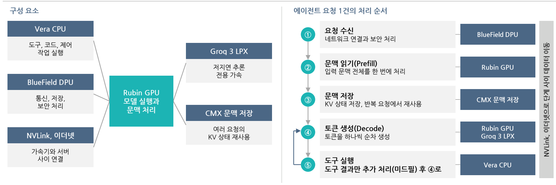
그림 26. 추론 시스템의 작업 분담
