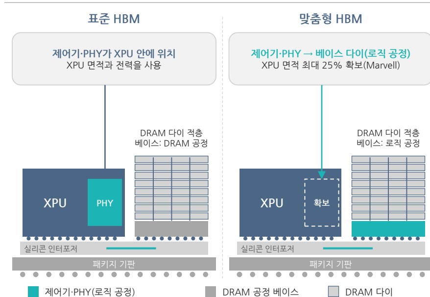
그림 37. 표준 HBM과 맞춤형 HBM의 패키지 단면
